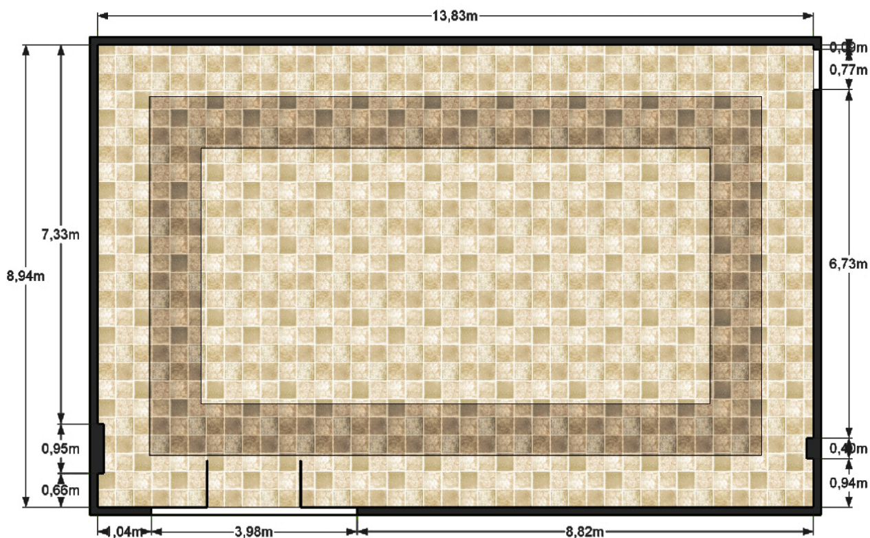
PLANTA BAIXA
